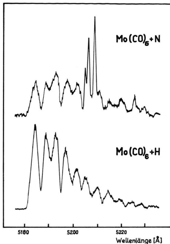
Abb. 1. Emissionsbande bei den Chemilumineszenzreaktionen Mo(CO)_6 + N und Mo(CO)_6 + H mit einer spektralen Auflösung von \Delta\lambda = 0,5 Å.
